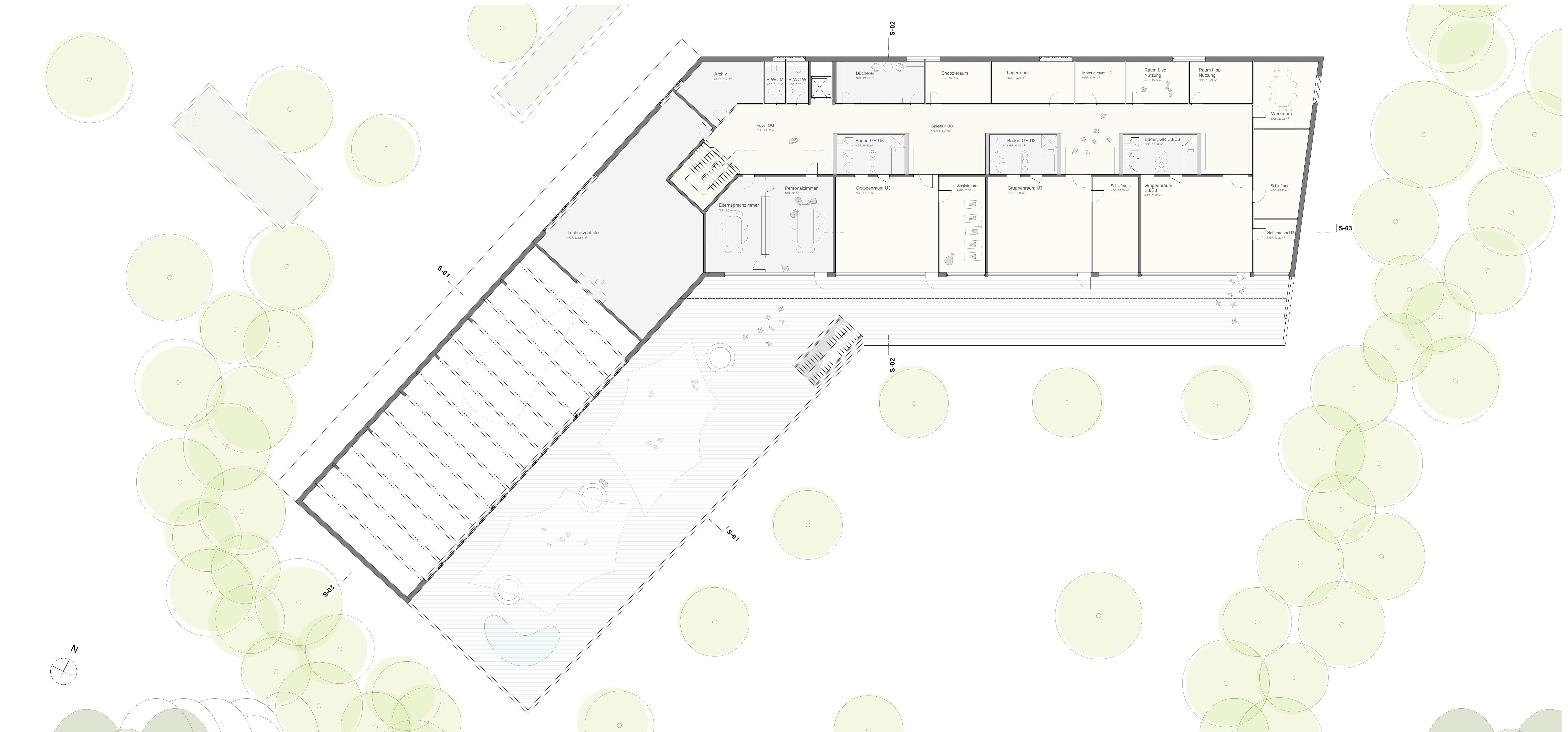
Grundriss OG 1:100 Schnitt 3 1:100
