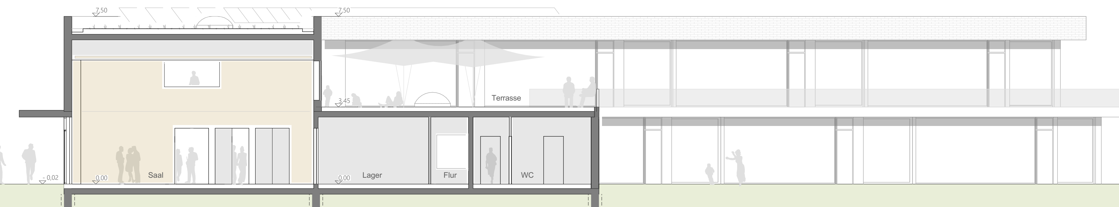
Schnitt 1 Quer 1:100
